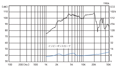
■周波数特性
