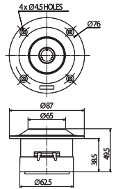
■寸法図
