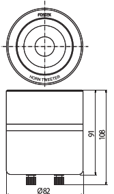
■寸法図
