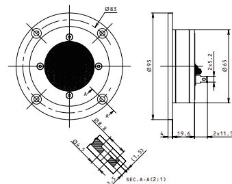
■寸法図
