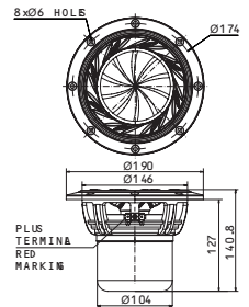
■寸法図
