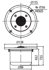
■寸法図
