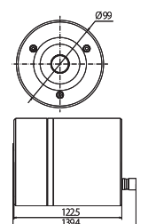
■寸法図
