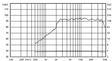
■周波数特性
