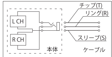
結線図
