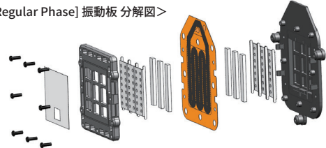
<RP [Regular Phase] 振動板 分解図>
