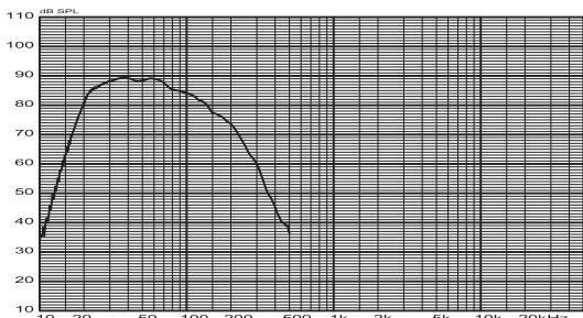
L.P.F. fc=90Hz特性
